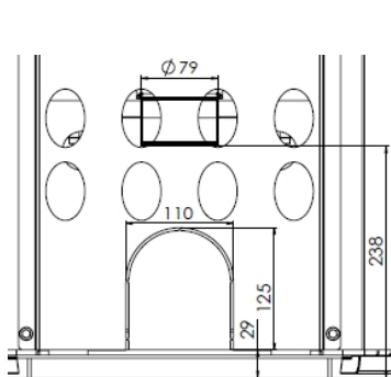
Montage mål Nordic 5 og 7 Air
