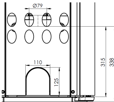
Montage mål Nordic 9 Air
