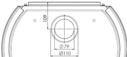
Montage mål Nordic 5, 7 og 9 Air Set fra bunden
